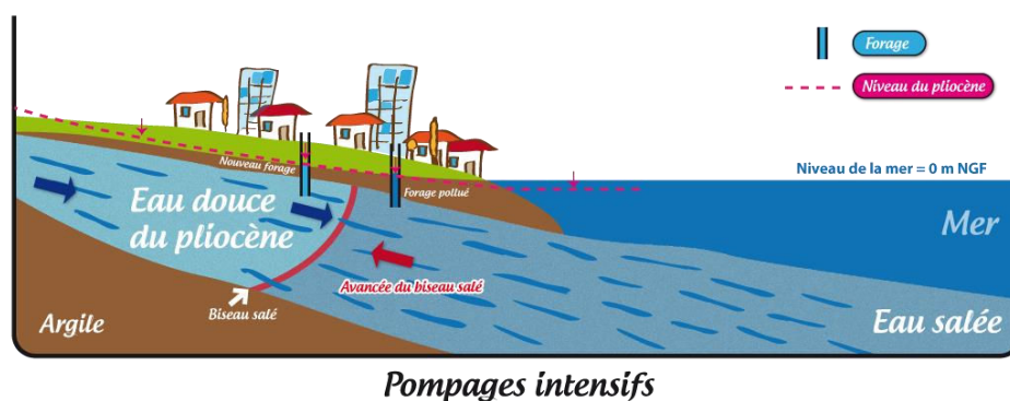
figure 3 : Schéma de principe de l'avancée du biseau salé
