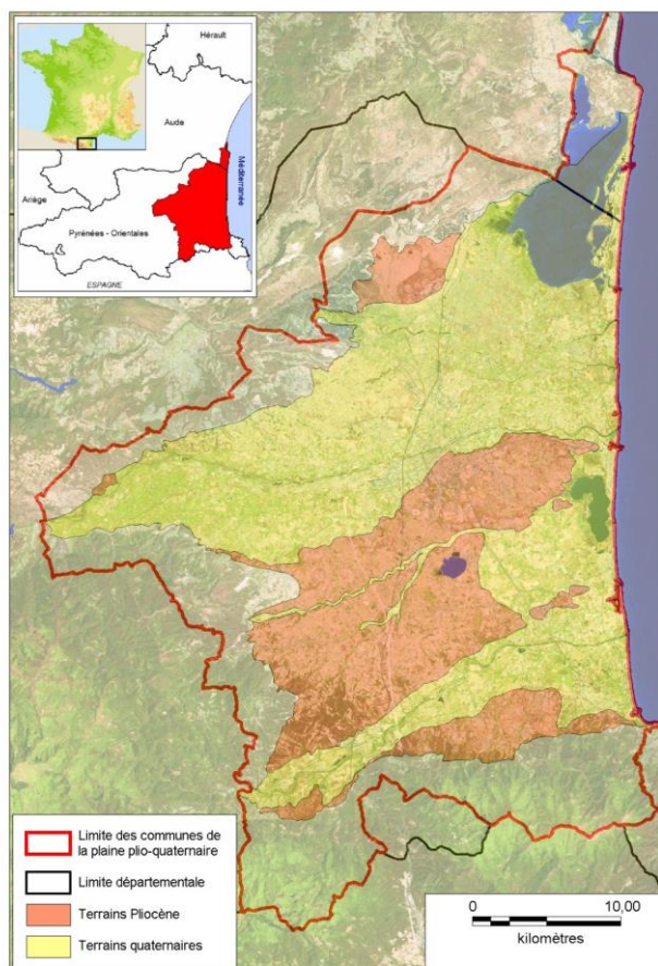
figure 2 : Cartographie des terrains Plio-quaternaire sur la plaine du Roussillon
