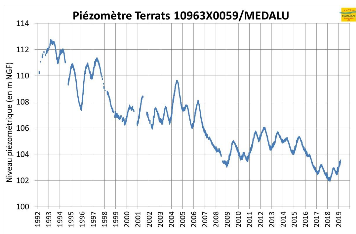
figure 4 : Evolution de la piézométrie à Terrats depuis 1992
